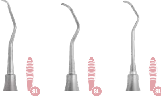
627/2.HL8 627/2.SL Columbia 2R/2L Anterior 627/4.HL8 627/4.SL Columbia 4R/4L Posterior 627/14.HL8 627/14.SL Columbia 13/14 Posterior
